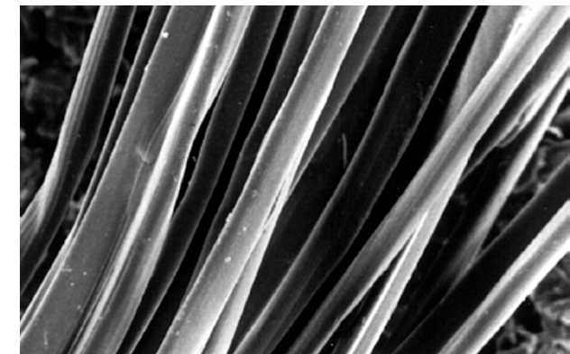
Abbildung: Längsansicht von Seidenfasern. Die Maulbeerspinnerseide weist eine glatte Oberfläche mit Verdickungen und fibrillären Abspaltungen auf (REM-Aufnahme Hohenstein Institute).
